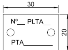
Figura 22. Identificación fusibles.
