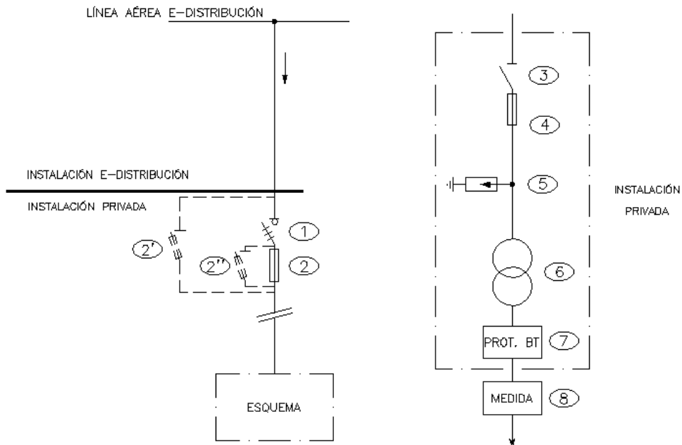
TIPO ACOMETIDA 1
