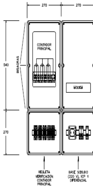
Figura 3. Conjunto modular
