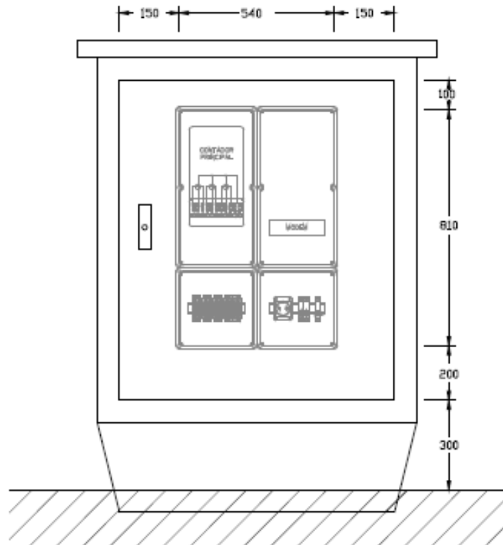
Figura 4. Armario modular
