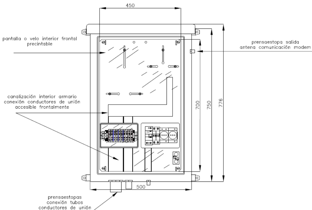
Figura 2. Armario
