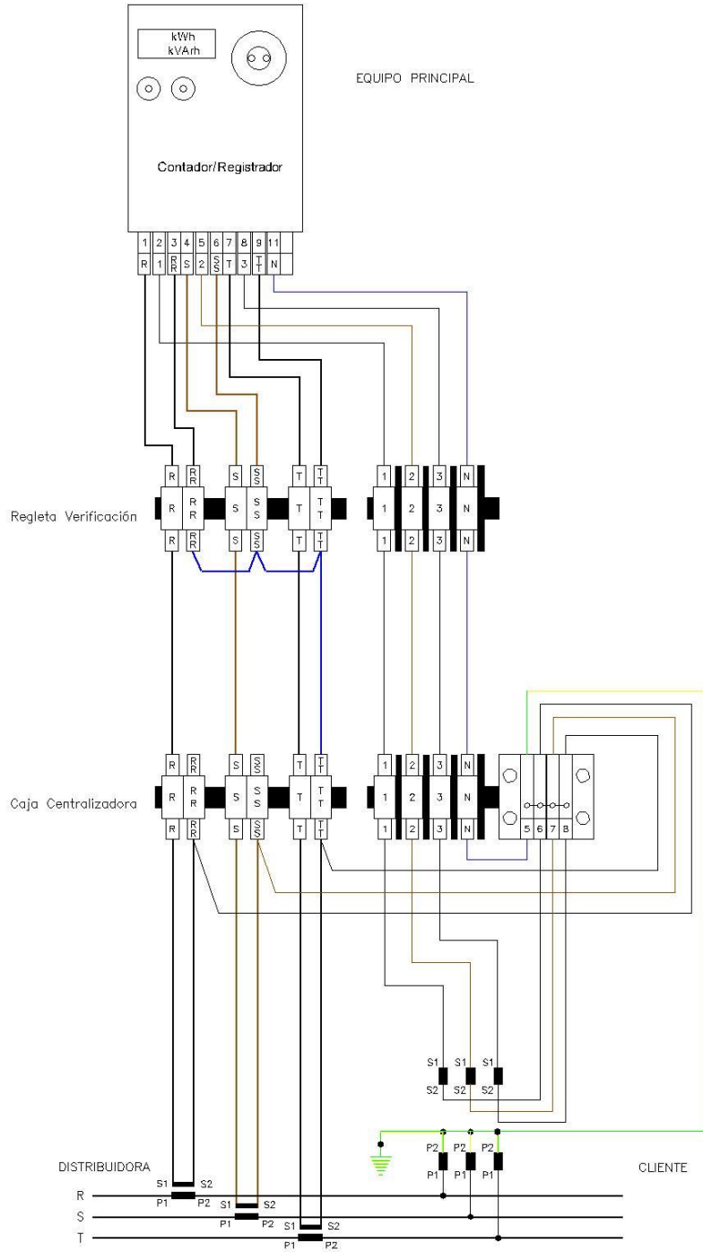
Figura 6. Esquema de conexonado con caja centralizadora
