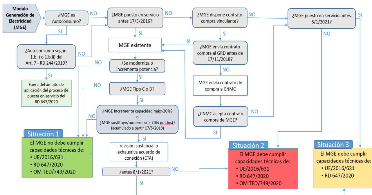
Figura 1 - Flujograma – Condiciones para determinar las capacidades técnicas para los MGE conectados a la RdD del sistema eléctrico peninsular.
